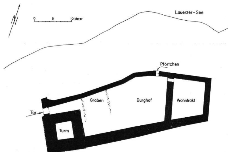
Abb. 1: Grundriss der Schwanau nach der Ausgrabung 1960. Quelle: Nachrichten des Schweizerischen Burgenvereins, Band 33 (1960)
